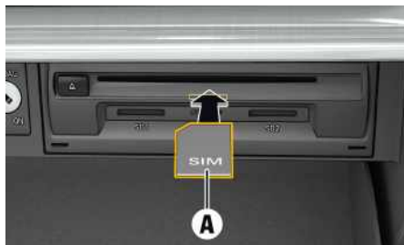
Fig. 1: Insertion et retrait d'une carte SIM
